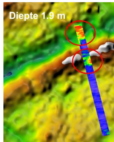
De smalle strook van de meting toont sterke (rode) reflecties van de muur (onder) en de greppel (boven).
