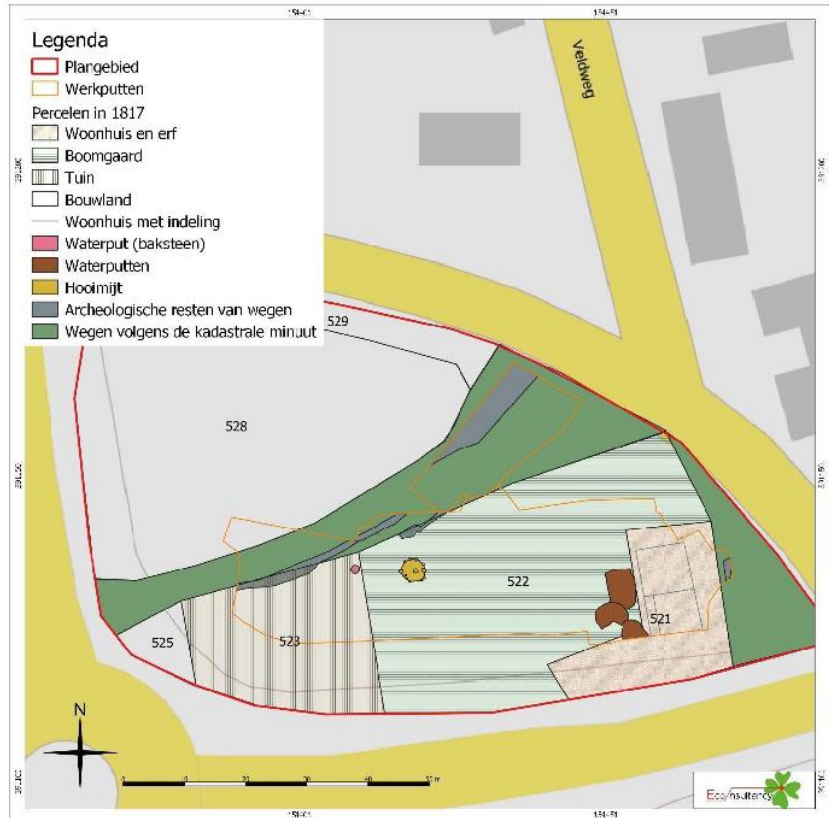
Overzicht indeling volgens de kadastrale minuut uit 1817 gecombineerd met de archeologische resten van het boeren erf.
