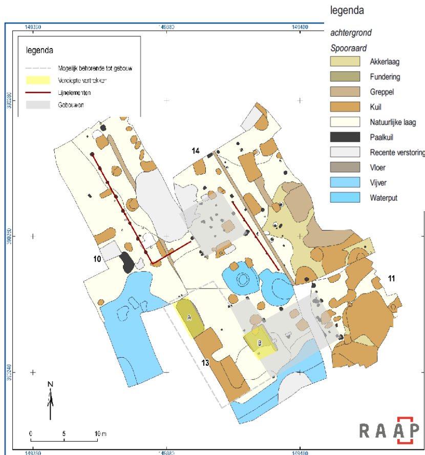
Structuren op de allesporenkaart met werkputnummers
