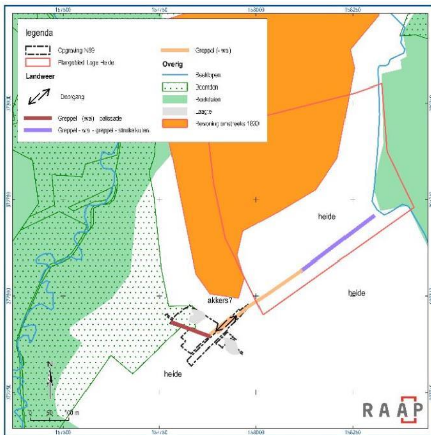
Figuur 130. Schematische weergave van de landweer tussen de Keersop en de Oude Dommel. Schaal 1:7000.
