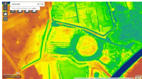
Ter Borch – Oisterwijk: voormalig grachtenstelsel en andere relictten op de AHN-kaart.
