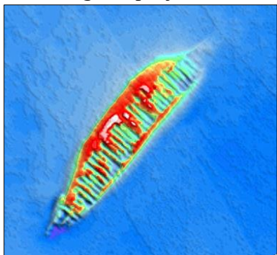
Sonar van de KR 321
